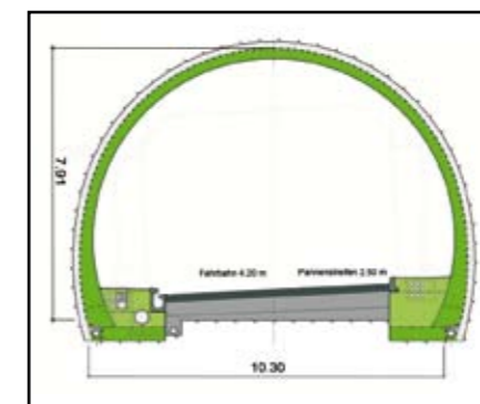
Normalprofil des Überwurf tunnels
