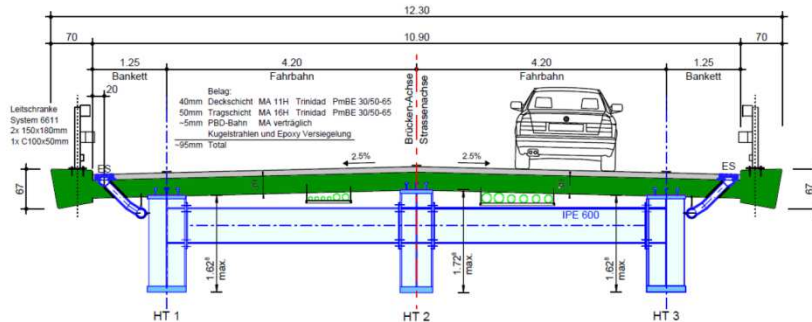
QUERSCHNITT 1:100
