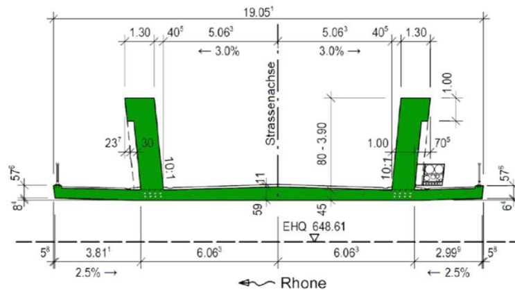
Schnitt A-A
